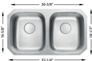
S-DEB202-16H S-DEB202-18H Depth 9" Depth 9" 16 Gauge 18 Gauge
